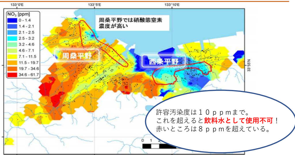
図 2-12 地下水の硝酸態窒素濃度の分布
